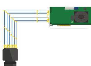
1台の8接続 カメラ
