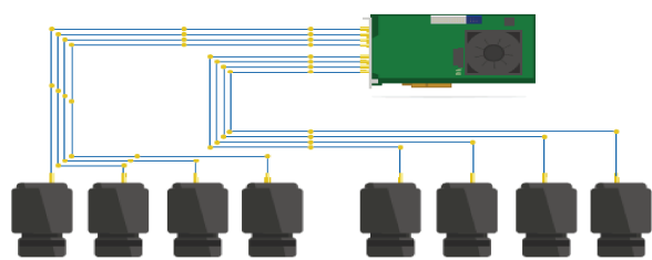
8台の1接続 カメラ
